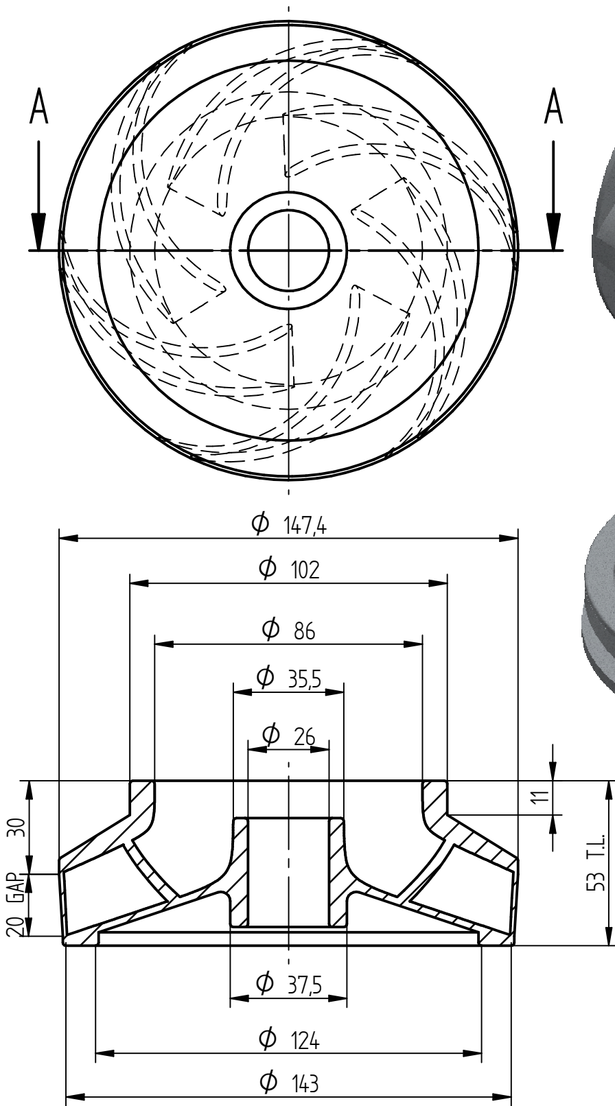
SECTION A-A
