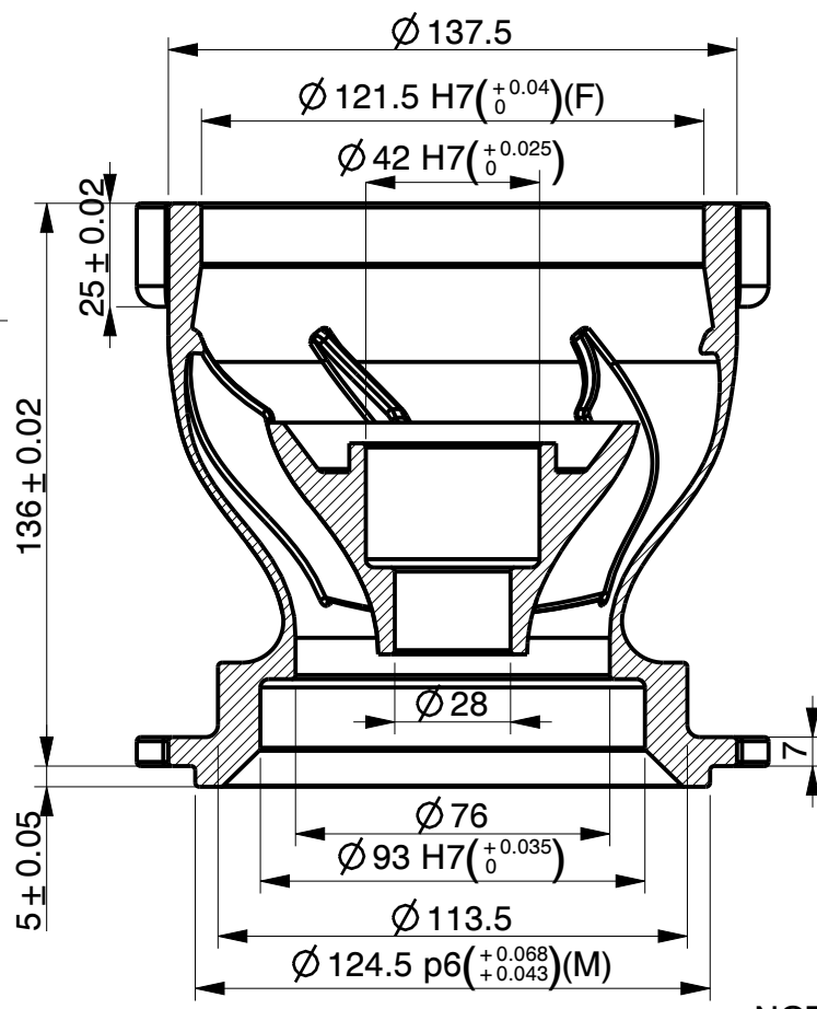
SECTION A-A
