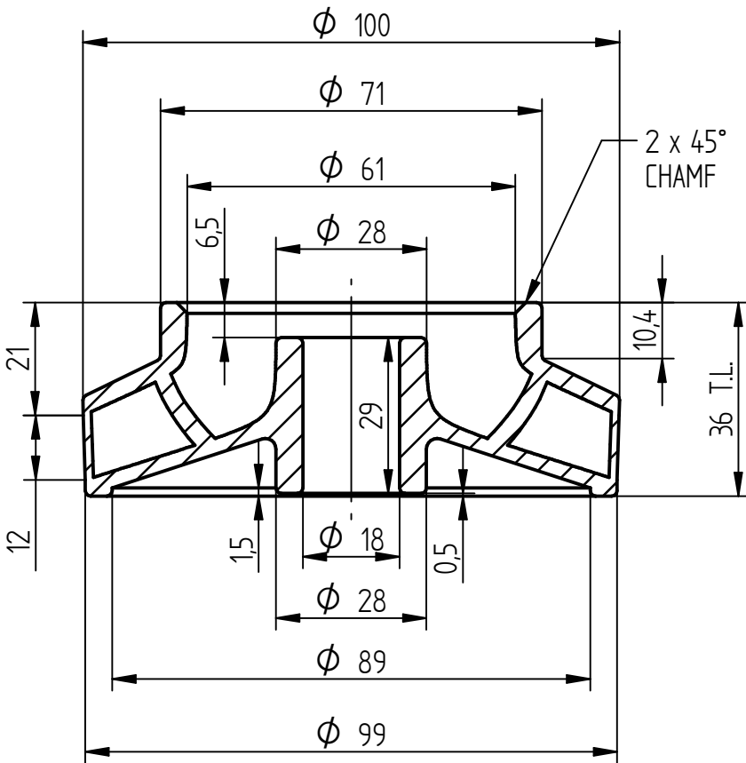
SECTION A-A
