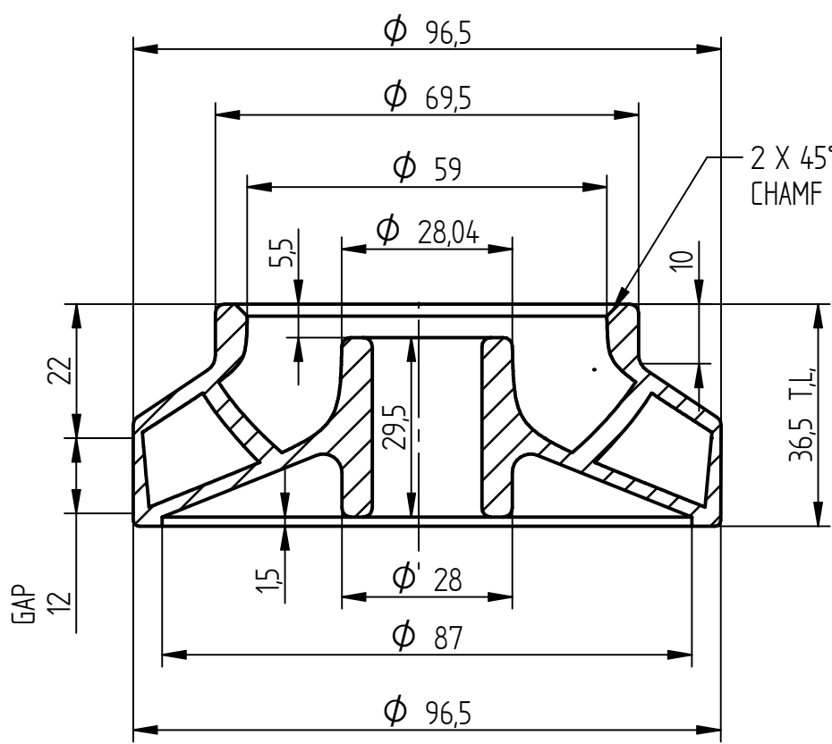
SECTION A-A
